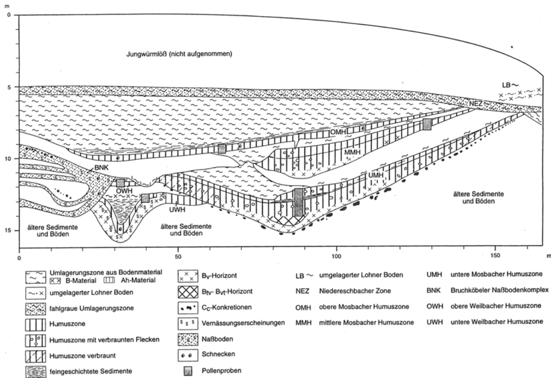
Abb. 18. Horizontabfolge des Altwürmlössabschnittes in Dellenposition (aus Bibus et al., 1996).
