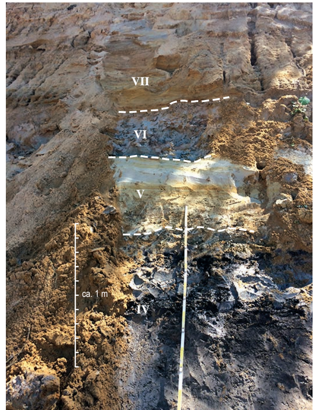
Abb. 9. Ausschnitt aus der Sedimentabfolge der Tongrube am Katzenbuckel. Die einzelnen Profilabschnitte beschreiben: IV = limnisch-fluviatile, holzführende Torfe und stark humose Tone; V = stark gebleichte, glimmerführende, fluviatile Sande; VI = limnisch-fluviatile, schluffige Tone und VII = oxidierte, fluviatile Mittel- bis Grobsande. (Foto: Christian Hoselmann)
