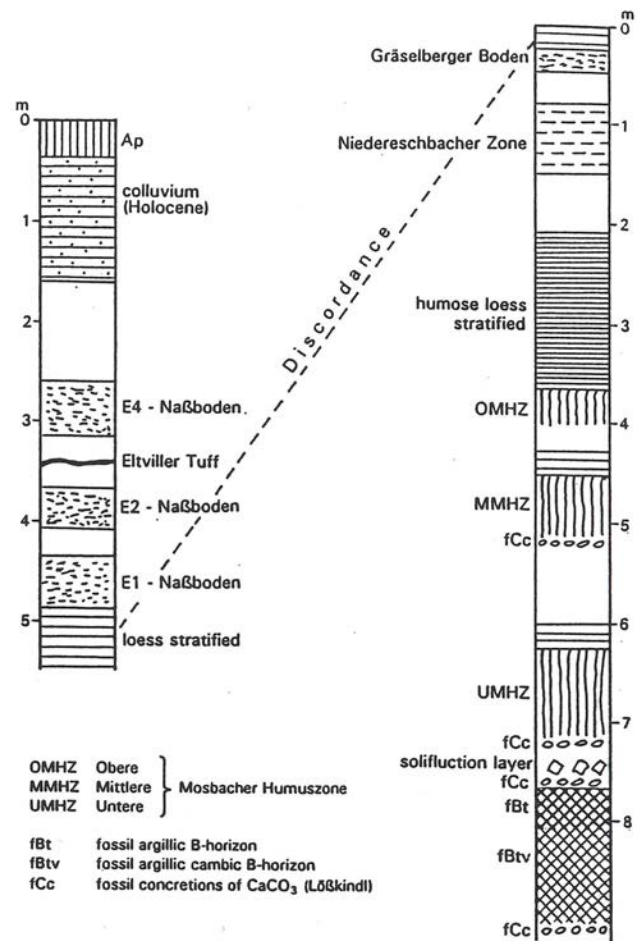
Abb. 17. Würmlössprofil in Mainz-Weisenau aus Semmel (1999c).
