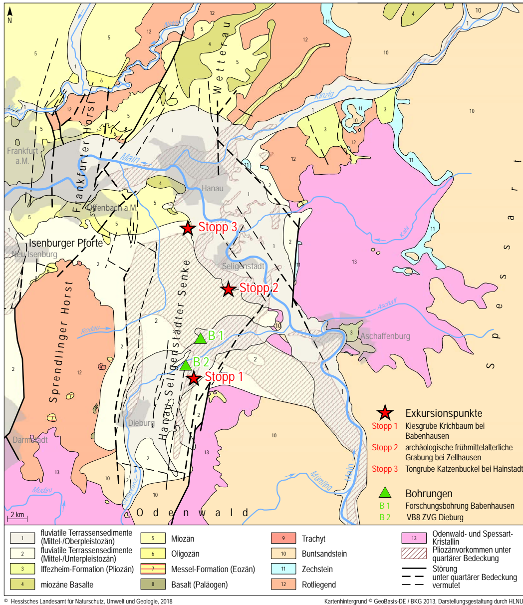
Abb. 3. Geologische Übersichtskarte des östlichen Rhein-Main-Gebietes (verändert nach Lang und Seidenschwann, 2012).
