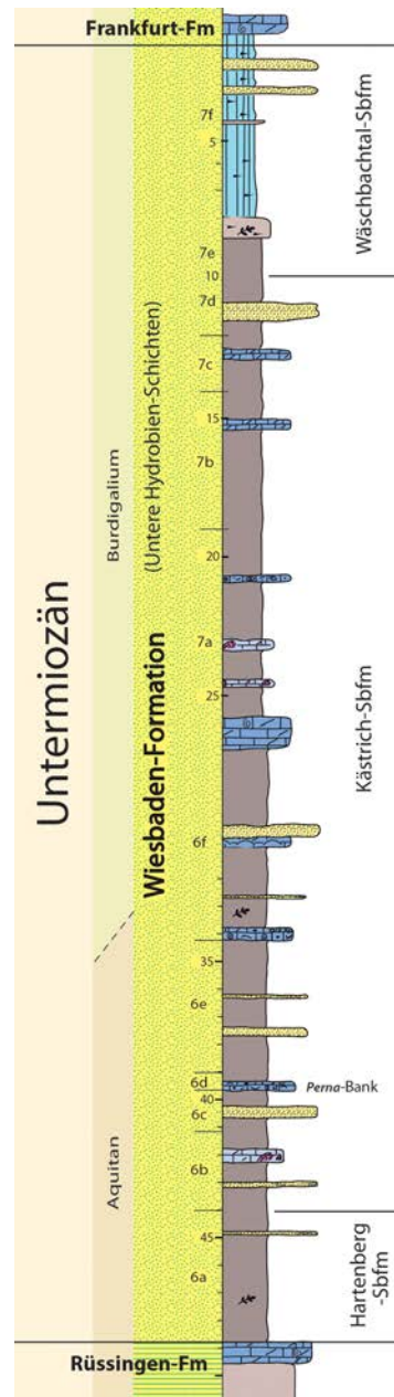
Abb. 11. Standardprofil der Wiesbaden-Fm mit Subformationen (nach Radtke, 2007, verändert).
