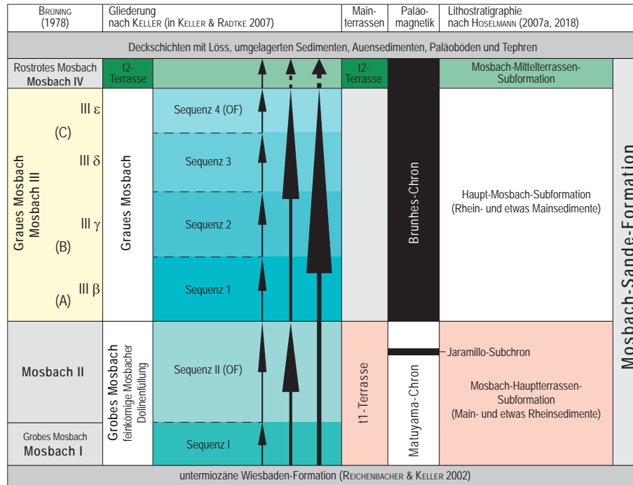
Abb. 14. Schematische Untergliederung der Mosbacher Sande (umgezeichnet nach Keller in Keller und Radtke, 2007) mit einer zyklthemischen Gliederung (kurze Pfeile: Kleinzyklen – längere Pfeile: übergeordnete Zyklen – OF = Overbank-Fine); im Grauen Mosbach werden vier Sequenzen nachgewiesen, die einzelnen Flussarchitekturen: (1) verflochtener Fluss, (2) mäandrierend sandige Mischform, (3) schmale anastomisierende Rinnen und (4) Overbank-Fines, zugerechnet werden. Ergänzt wird diese Darstellung durch die paläomagnetische Einstufung und um eine lithostratigraphische Neugliederung der Sedimentabfolge sowie die Gliederung des Aufschlusses nach Brüning (1978).
