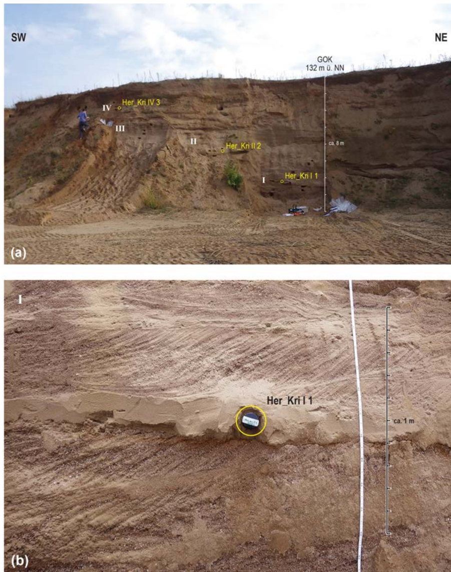
Abb. 5. (a) Übersichtsfoto der Abbauwand in der Kiesgrube Krichbaum bei Babenhausen – in dem Foto sind die vier Profilabschnitte I–V sowie die Probenentnahmepunkte für die Lumineszenzdatierungen (Her_Kri I 1 etc.) vermerkt. (b) Detailausschnitt aus dem Profilabschnitt I mit schrägeschichteten fluviatilen Sedimenten der Gersprenz und dem Probenentnahmepunkt Her_Kri I 1 für die Lumineszenzdatierung (Fotos: Christian Hoselmann).
