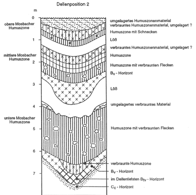
Abb. 20. Altwürmabfolge in Dellenposition, Profil Mainz-Weisenau (aus Bibus et al., 1996).
