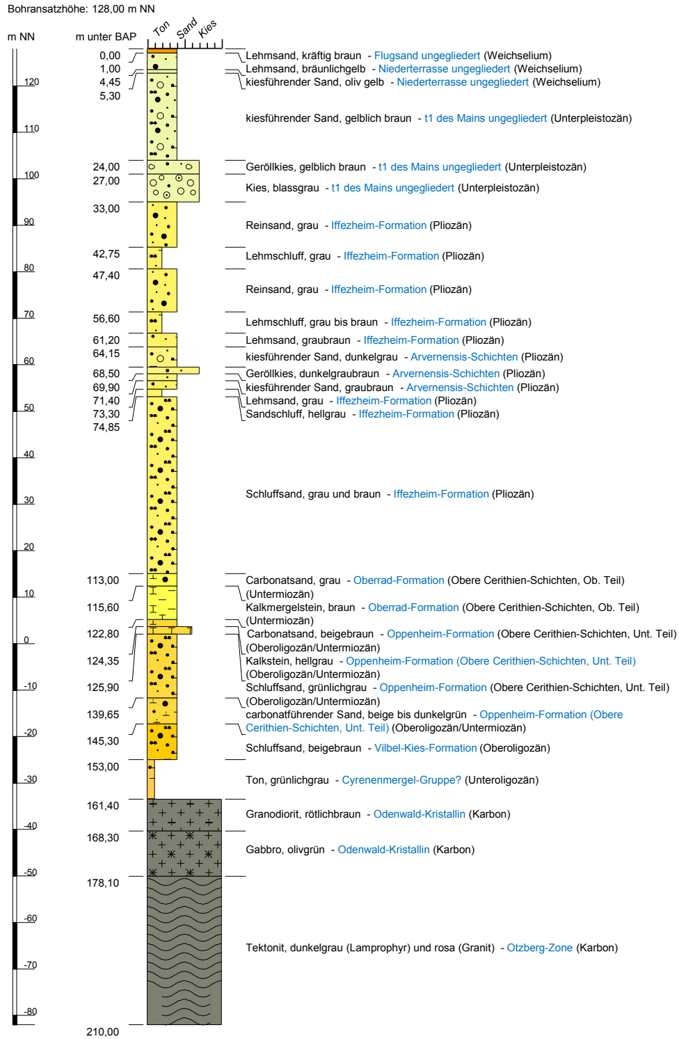
Abb. 4. Stark generalisiertes geologisches Profil der Forschungsbohrung nördlich von Babenhausen (R 3495591, H 5537260).
