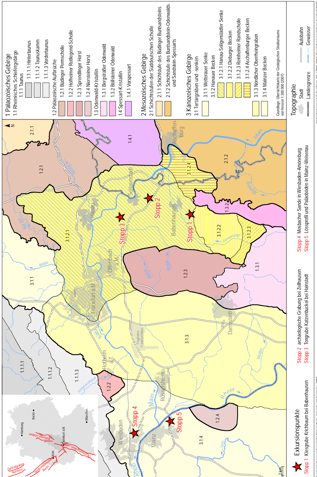
Abb. 1. Die geologischen Strukturräume im Exkursionsgebiet mit den einzelnen Stopps sowie den tektonischen Strukturen im westeuropäischen Riftsystem.
