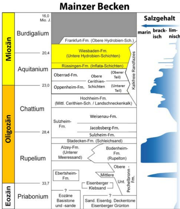
Abb. 10. Überblick zur Stratigraphie des Mainzer Becken mit Lage der marinen Ingressionen (nach Försterling und Radtke, 2012, verändert); in Gelb: aufgeschlossene Formationen im Dyckerhoff-Steinbruch.
